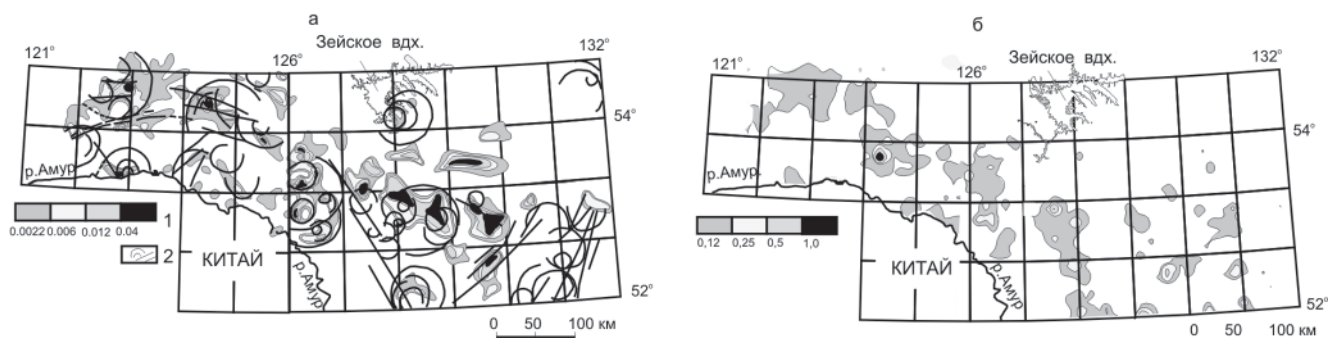
Рис. 2. Геохимические ореолы: а – золота по данным литохимических съемок по потокам рассеяния м-ба 1:200 000; б – серебра по данным литохимических съемок по потокам рассеяния м-бов 1:200 000–1:1 000 000
