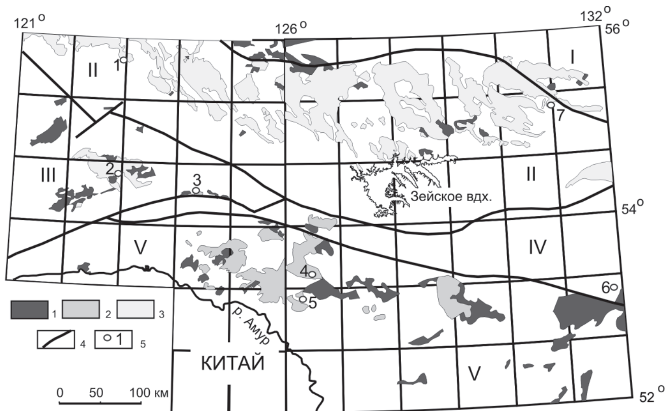
Рис. 1. Схема размещения вулканоплутонических и плутонических комплексов позднего мезозоя (по [5])
