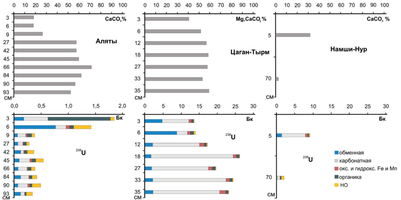
Рис. 2. Распределение по разрезу донных отложений озер Аляты, Цаган-Тырма и Намши-Нур кальция (в пересчете на CaCO 3 ) и 238 U по фракциям
